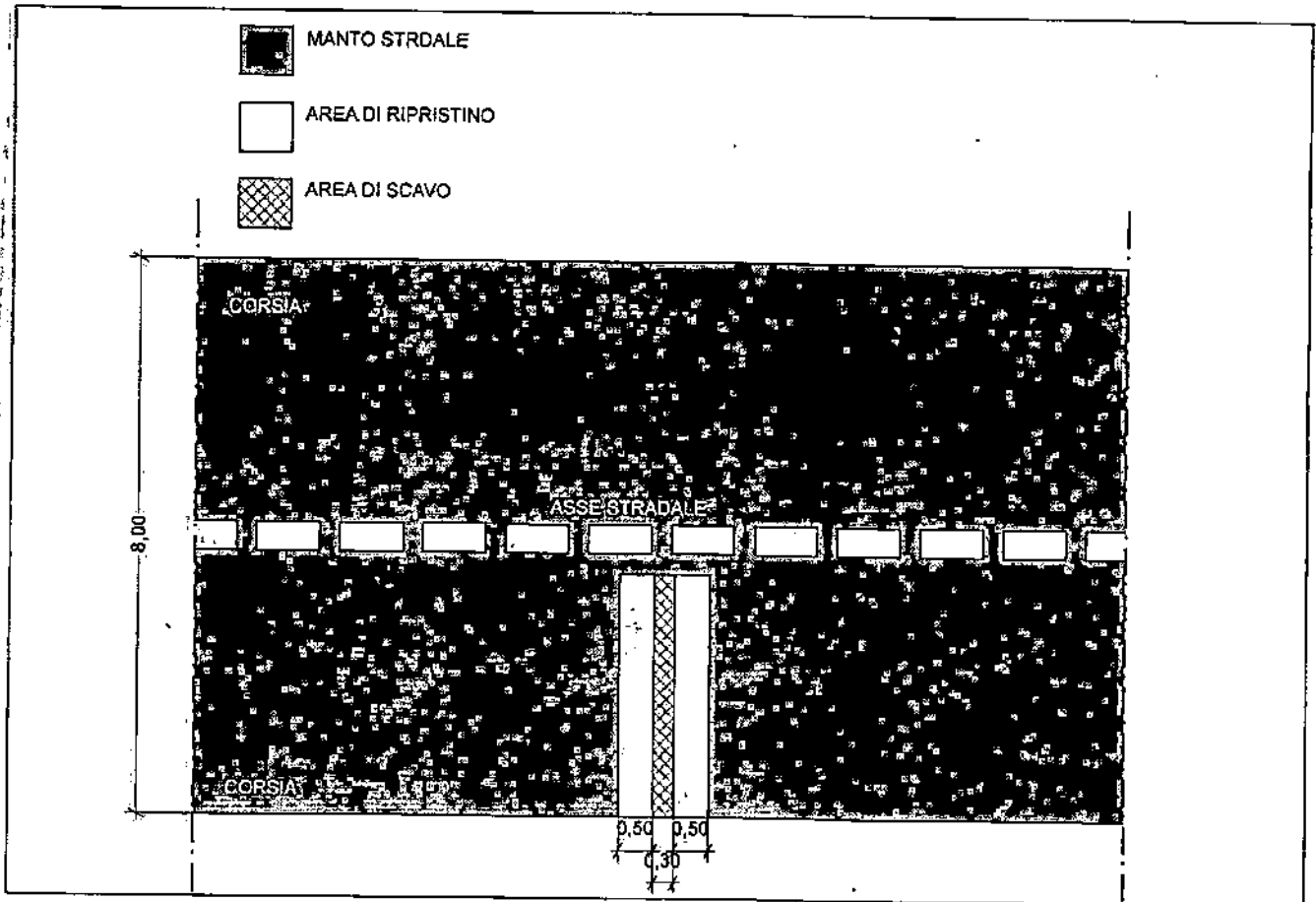
SCAVO TRASVERSALE ALLA CARREGGIATA
