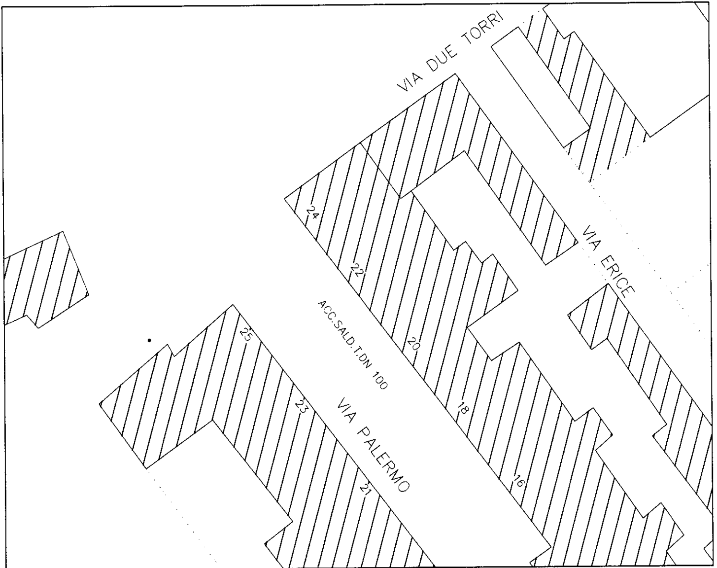
PLANIMETRIA SCALA 1:500
