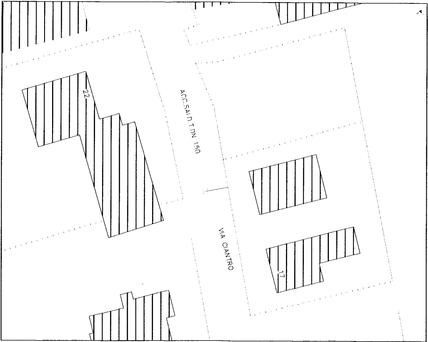
PLANIMETRIA SCALA 1:500
