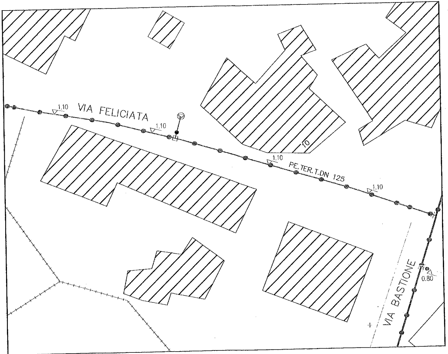
PLANIMETRIA SCALA 1:500
