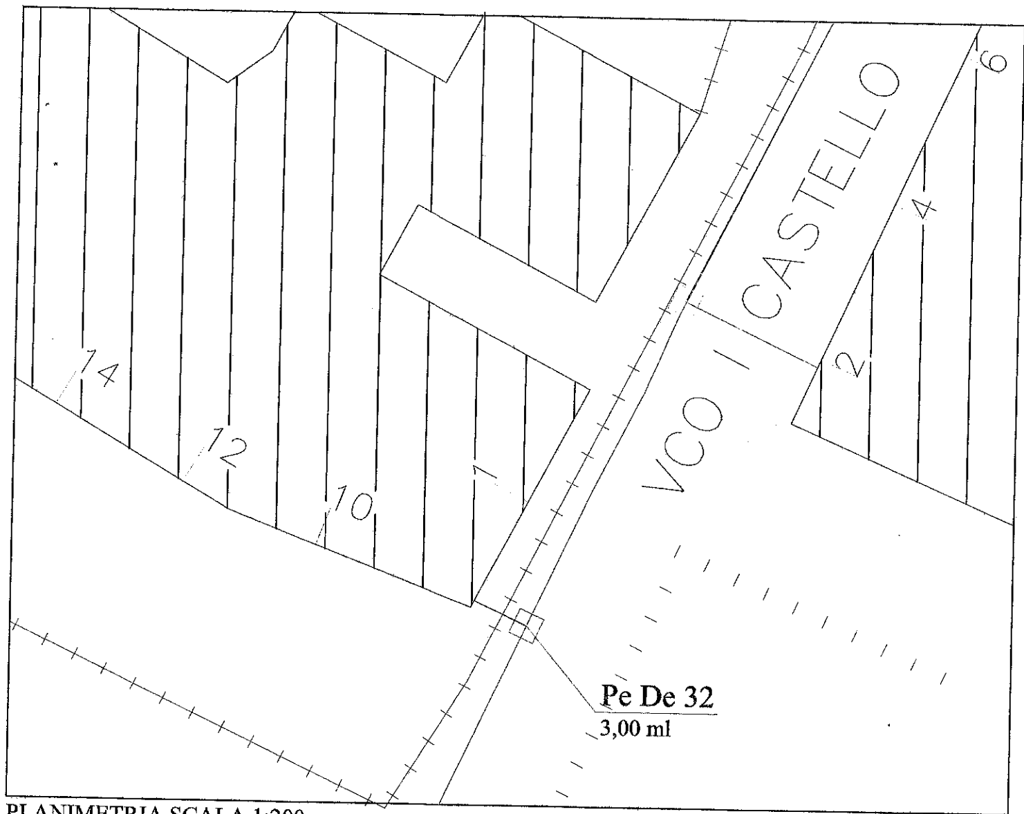
PLANIMETRIA SCALA 1:200
